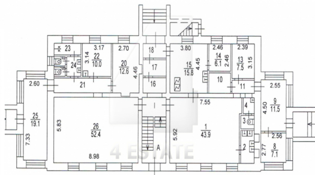
1 ЭТАЖ
