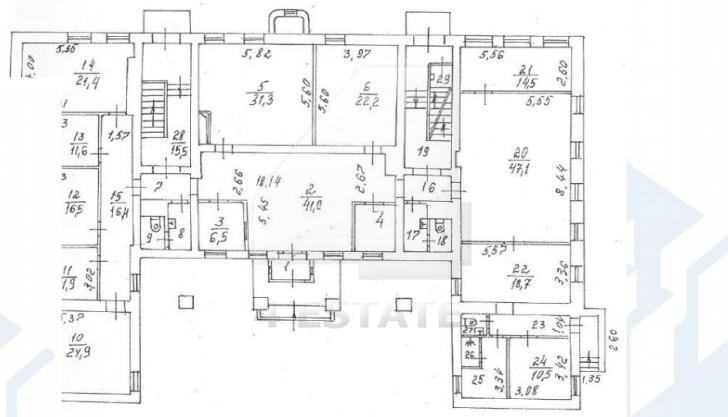
1 этаж
