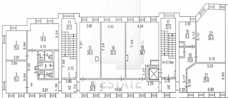
3 ЭТАЖ
