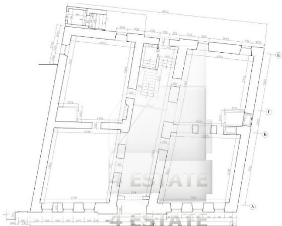
План 1-го этажа. Проект.
