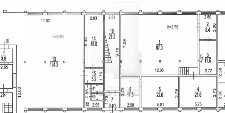
1 этаж(левое крыло)
