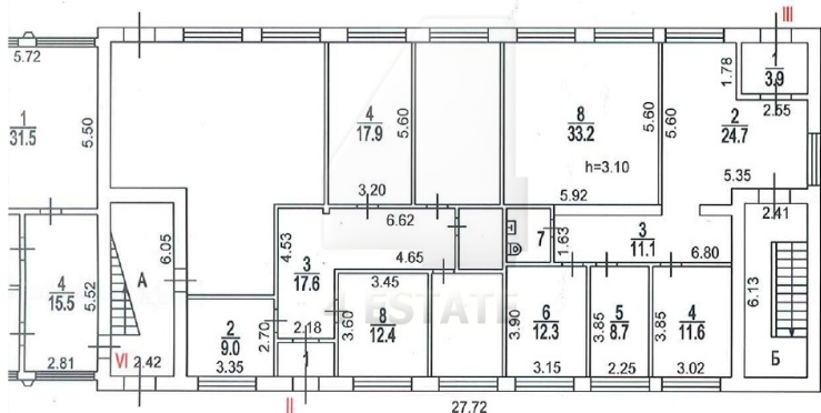
1 этаж(правое крыло)
