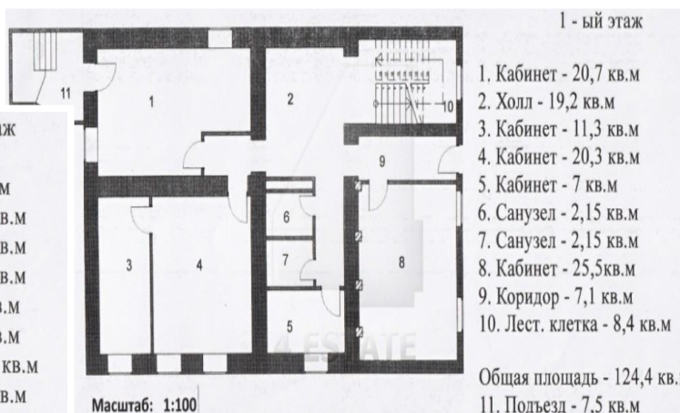
1 - ый этаж
