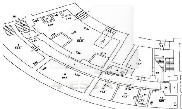
1 этаж антресоль
