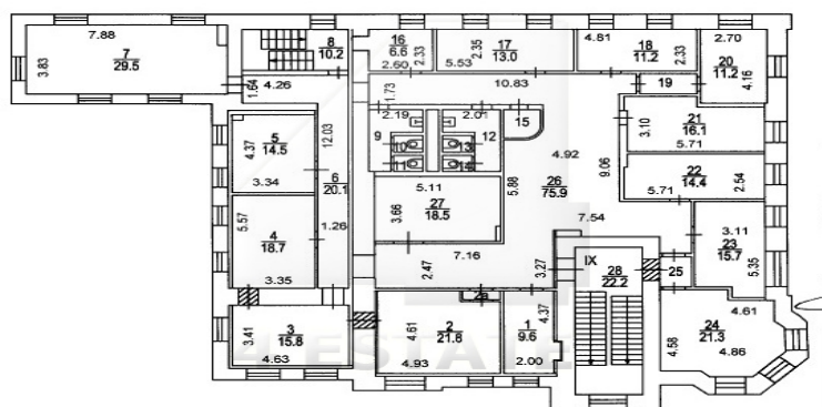
2 ЭТАЖ
