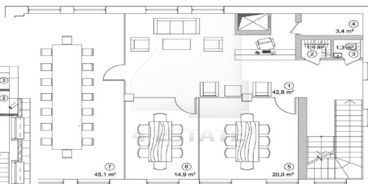
Второй этаж
