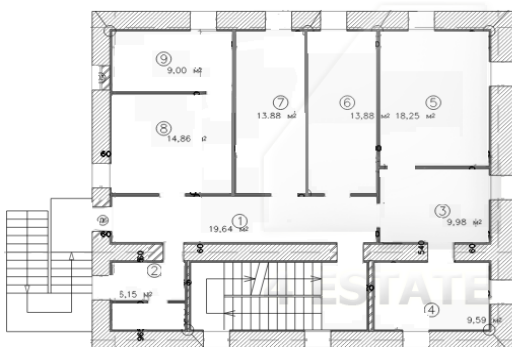
План мансарды
