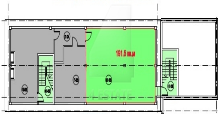
План подземного этажа на отм. -2.880
