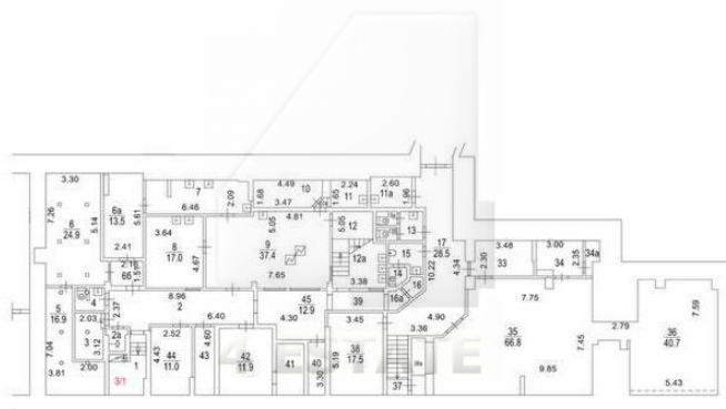
ПОДВАЛ
