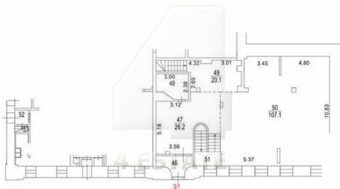
1 ЭТАЖ
