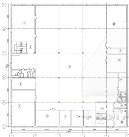
План 1 этажа
