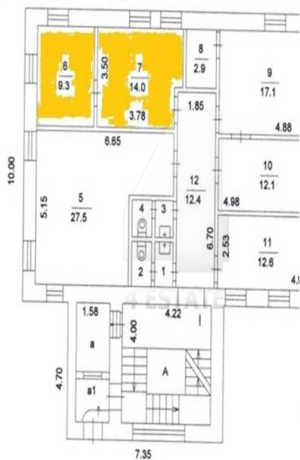
(1 этаж)
