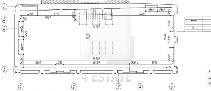
ОБМЕРНЫЙ ПЛАН ЧЕРДАКА М 1:100
