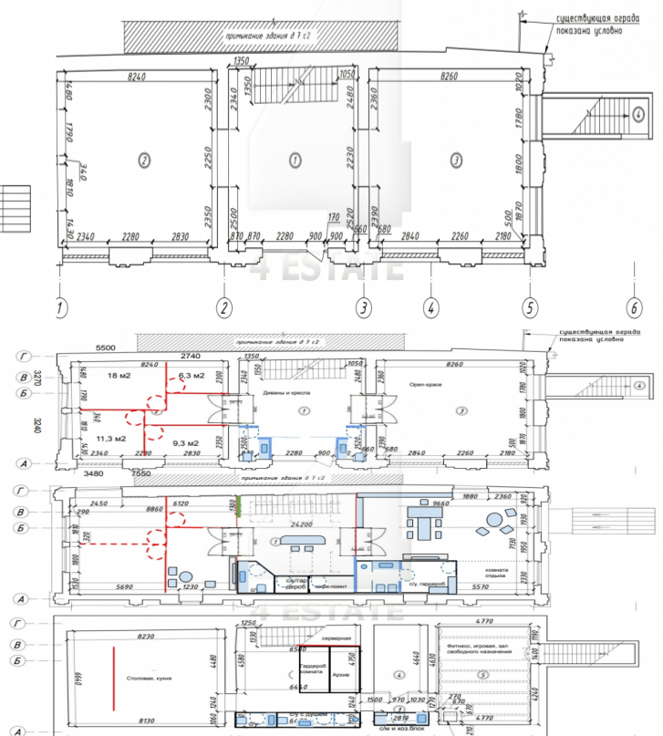
ОБМЕРНЫЙ ПЛАН 1-ГО ЭТАЖА М 1:100
