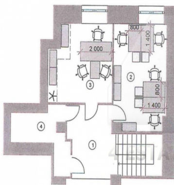
План антресольного этажа.
