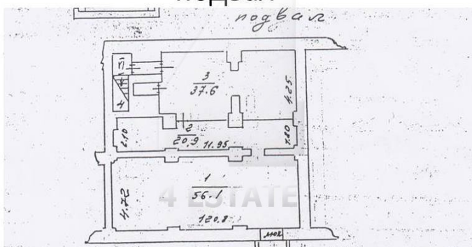
план схема подвал
