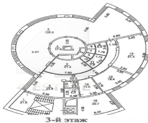
3-й этаж
