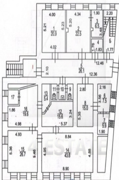
ЦОКОЛЬНЫЙ ЭТАЖ
