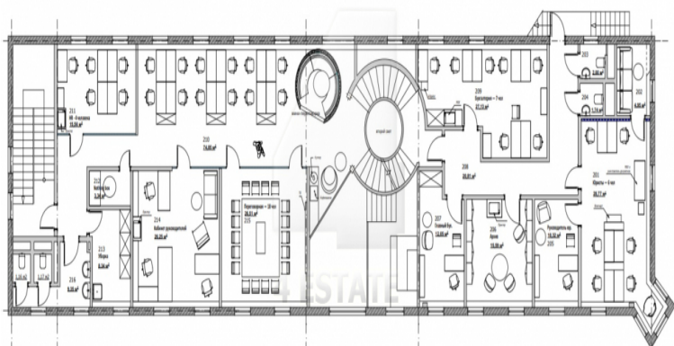
ПЛАН 2 ЭТАЖА С РАССТАНОВКОЙ МЕБЕЛИ И ОБОРУДОВАНИЯ
