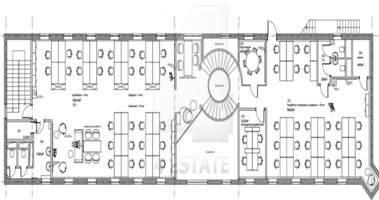
ПЛАН 3 ЭТАЖА С РАССТАНОВКОЙ МЕБЕЛИ И ОБОРУДОВАНИЯ
