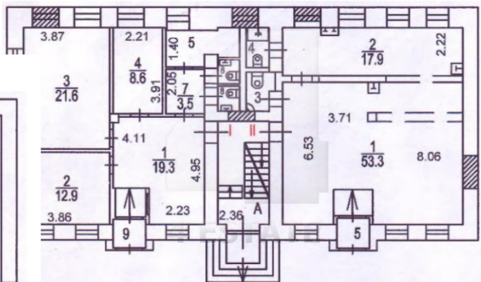
1й этаж:
