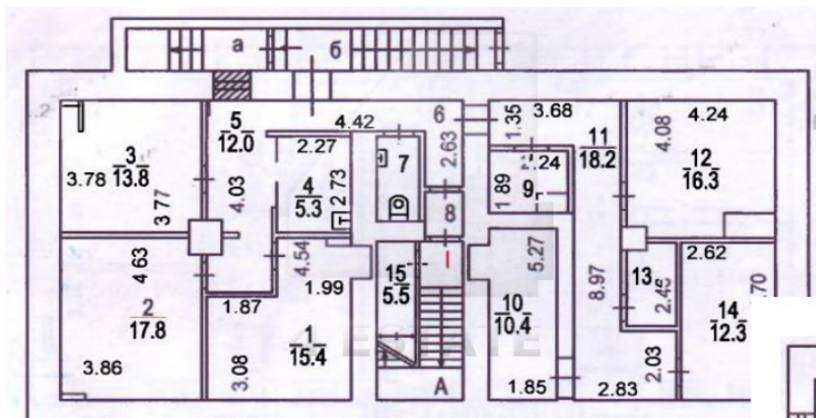
2й этаж:
