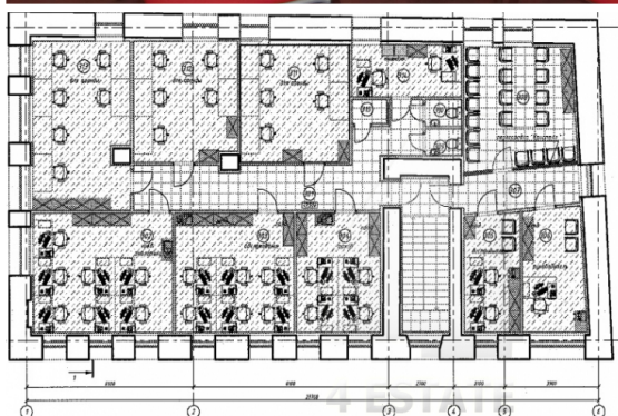
Экспликация помещений
