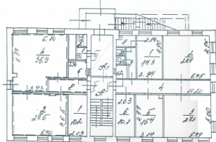
ПОДВАЛ
