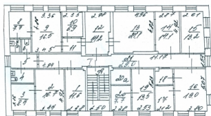
1 этаж
