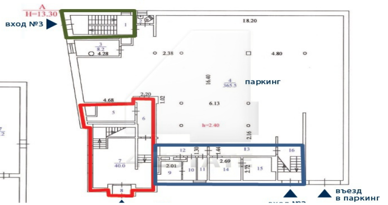
2 этаж
