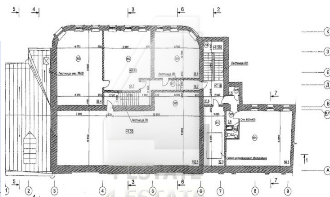
ПЛАН 1ого ЭТАЖА на отм. ±0.00 М 1:100
