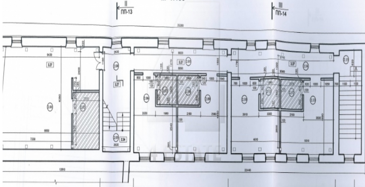
ПЛАН 2ого ЭТАЖА на отм. 3.90 М 1:100
