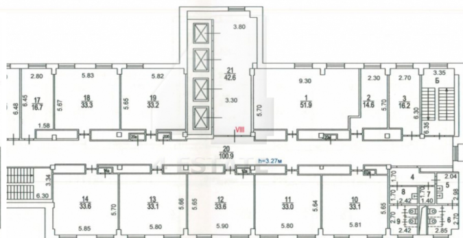
6 й ЭТАЖ
