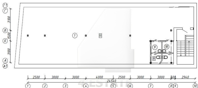
План эксплуатируемого чердака
