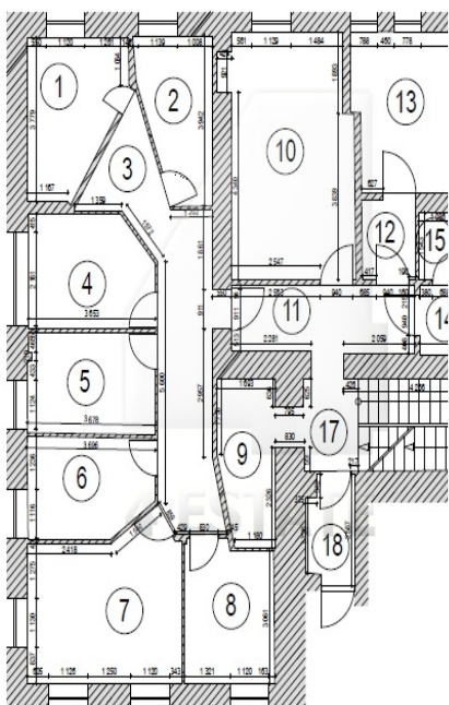
ПЕРВЫЙ ЭТАЖ
