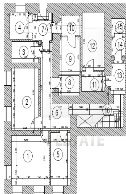
ЦОКОЛЬНЫЙ ЭТАЖ
