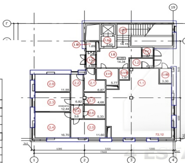
ЭКСПЛИКАЦИЯ ПОМЕЩЕНИЙ 2 ЭТАЖА
