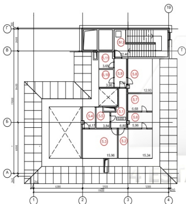
ЭКСПЛИКАЦИЯ ПОМЕЩЕНИЙ АНТРЕСОЛЬНОГО ЭТАЖА
