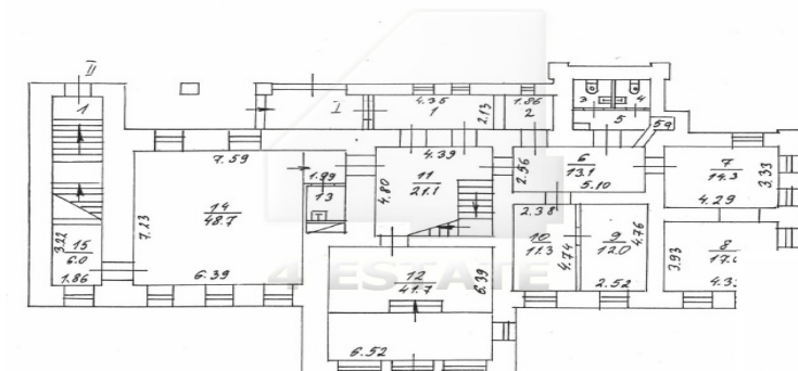
1 И ЭТАЖ
