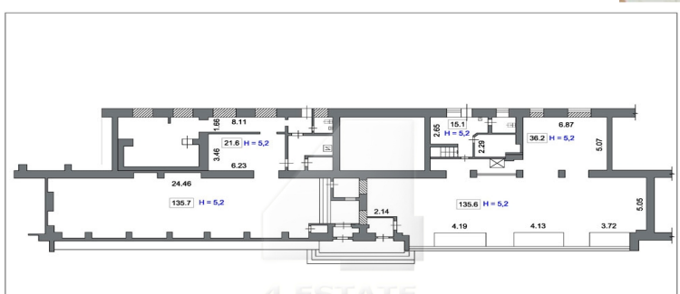
1-й ЭТАЖ м 1 : 200 Общая площадь 340,0 кв.м
