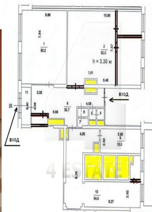
План Схема помещений офиса № 18
