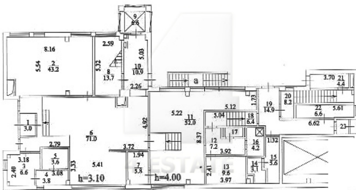
План 2 этажа
